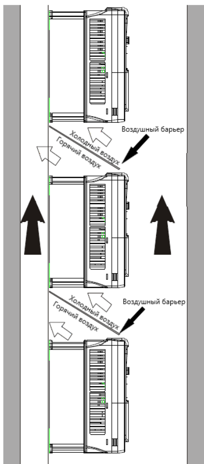
Рис. 4-5 Вертикальная установка
